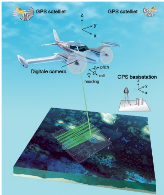
Figuur 20.5 Inwinningstechniek ALS (Bron: USGS)
