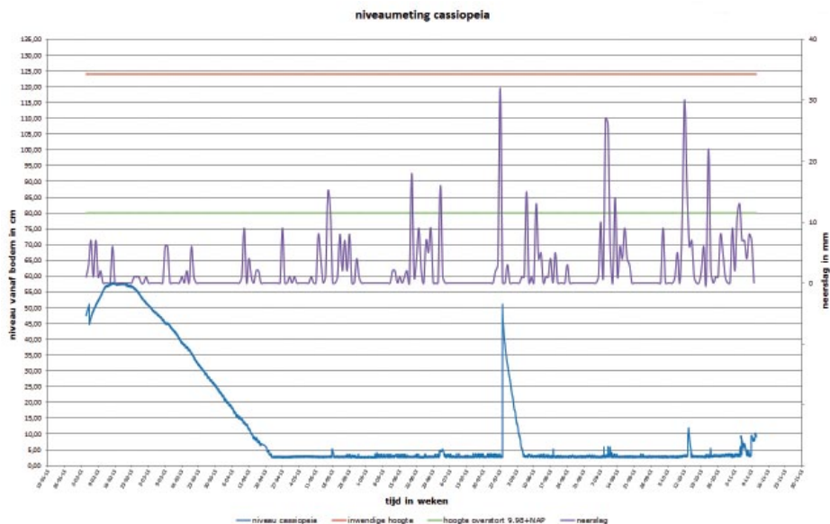
Figuur 2.12 Meetgrafiek bergings- en infiltratiekelder Cassiopeia.
