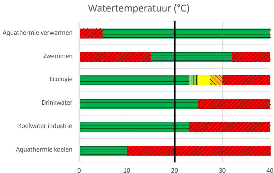
Figuur 3 Indicator watertemperatuur met functies die door watertemperatuur beïnvloed worden. Groen (horizontaal gearceerd) geeft aan dat de functie goed vervuld kan worden met betrekking tot watertemperatuur. Rood (schuin naar boven gearceerd) dat de functie niet of slecht vervuld wordt en lichtgroen, geel, oranje zitten daar tussenin. In dit voorbeeld is de huidige watertemperatuur 20 °C. Klimaatverandering leidt tot een hogere watertemperatuur. Als in de zomer de watertemperatuur \geq 23 °C wordt, is dit nadelig voor de functie koelwater. Bij een nog iets hogere temperatuur (25 °C) komt de drinkwaterwinning in gevaar en boven de 32 °C is het water minder geschikt voor zwemmen.
