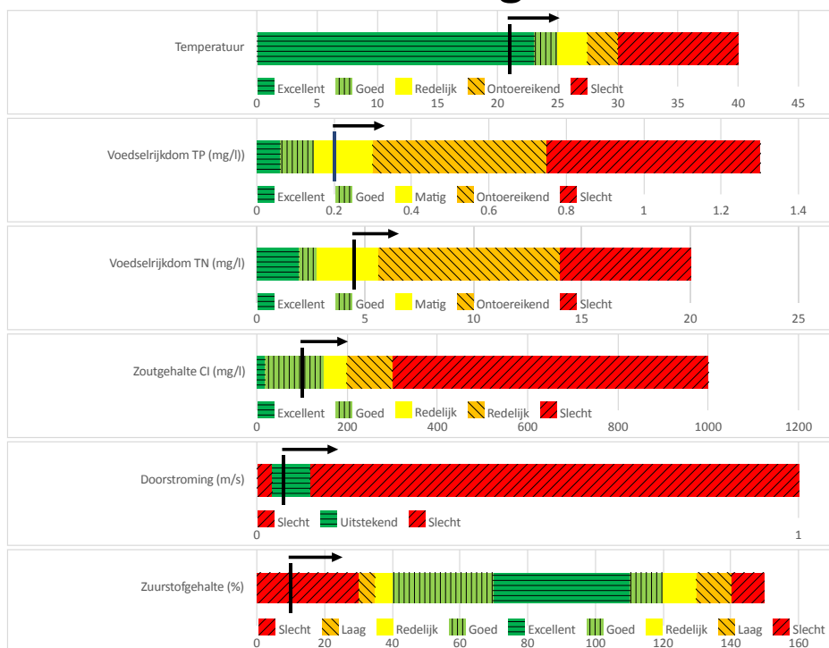
Figuur 4 Functie Ecologie voor een M3 watertype (brede sloot) met indicatoren die de functie beïnvloeden. De zwarte streep geeft de huidige toestand aan, de pijl de richting waarop de waarde van de indicator zal veranderen met klimaatverandering en de kleuren in de balk tussen welke waarden de indicator slecht, redelijk, goed of excellent is voor de functie Ecologie. De figuur laat voor de functie Ecologie van een brede sloot (watertype M3) zien welke indicatoren invloed hebben op deze functie. Naast elke indicator staat een horizontale balk. De zwarte streep op de balk geeft de huidige toestand van de indicator aan. De pijl geeft aan in welke richting de waarde van de indicator zal veranderen met klimaatverandering. De kleuren en patronen op de balk geven aan bij welke waarden een indicator een positief of negatief effect heeft op de ecologie van een brede sloot. Daarbij is donkergroen met horizontale arcering Excellent, lichtgroen met verticale arcering Goed, geel zonder arcering Redelijk, oranje met arcering schuin naar beneden Ontoereikend en rood met arcering schuin omhoog Slecht.
