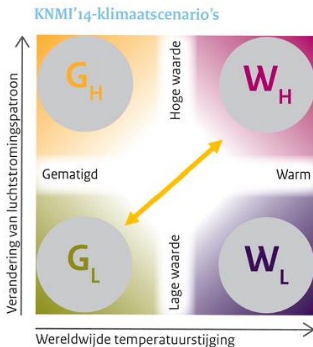
Figuur 4 KNMI'14 Klimaatscenario's
