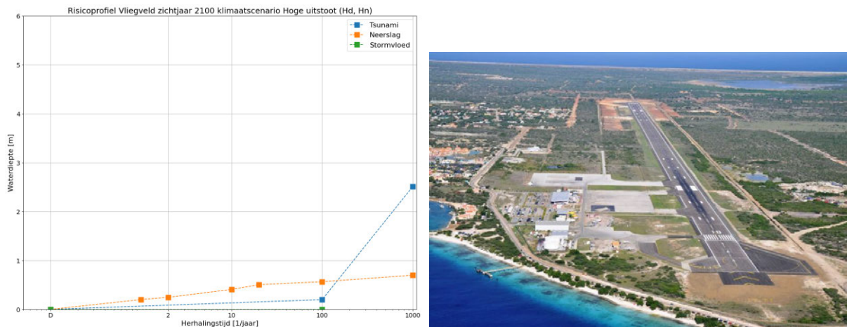
Figuur 23: Waterrisicoprofiel voor het vliegveld van Bonaire voor zichtjaar 2100 en hoge uitstoot scenario (links) en een foto 4 van de locatie (rechts). Vliegveld is ook bij een zeespiegelstijging van 85 cm niet kwetsbaar voor een stormvloed. Wel voor wateroverlast door regenval. Diepe inundatie kan alleen optreden in geval van een Tsunami, waarvan de kans wordt ingeschat als erg klein (1/1000).
