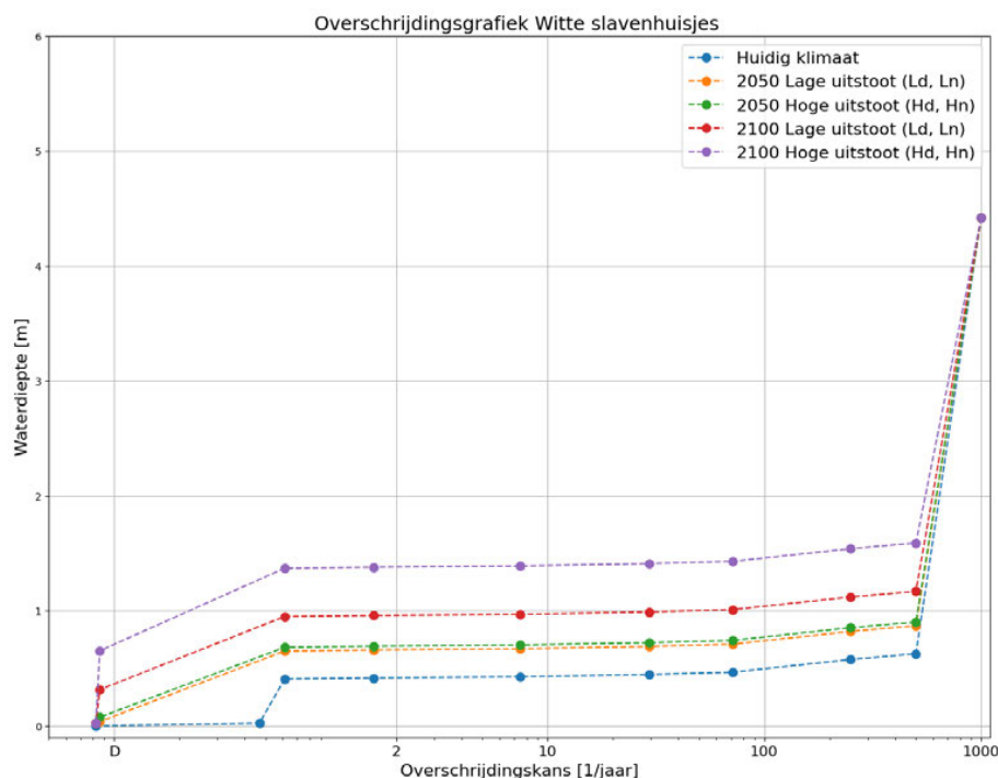
Figuur 24: Waterrisicoprofiel voor alle zichtjaren en type overstromingen voor de locatie witte slavenhuisjes. Hierin is te zien dat de witte slavenhuisje al bij een dagelijkse situatie overstromen door zeespiegelstijging. Bij gebeurtenissen tussen de eens per jaar en eens per 1000 jaar varieert de waterdiepte tussen een halve meter en 1,5 meter afhankelijk van het zichtjaar en klimaatscenario. Bij een tsunami (eens per 1000 jaar) zal de waterdiepte nog verder toenemen.
