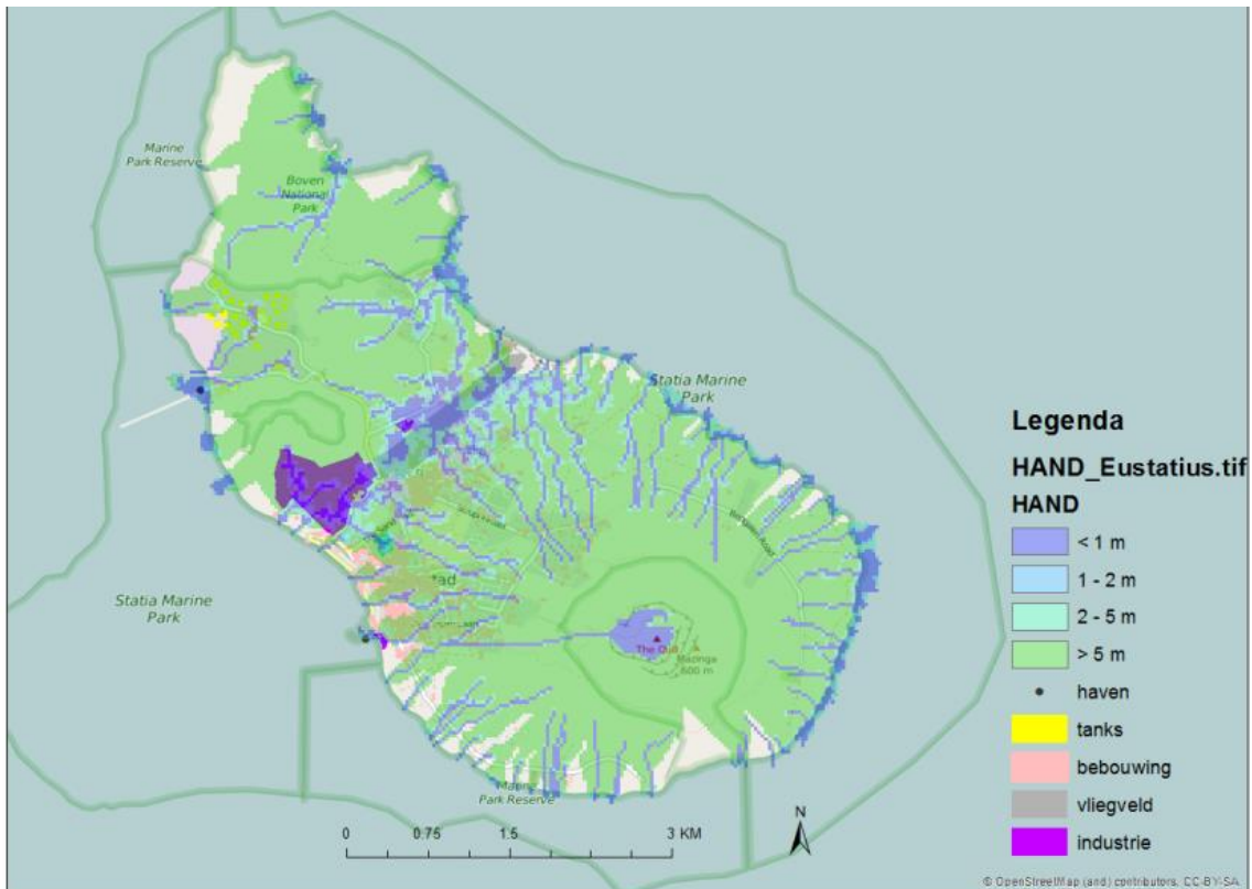
Figuur 36: HAND index Sint Eustatius.
