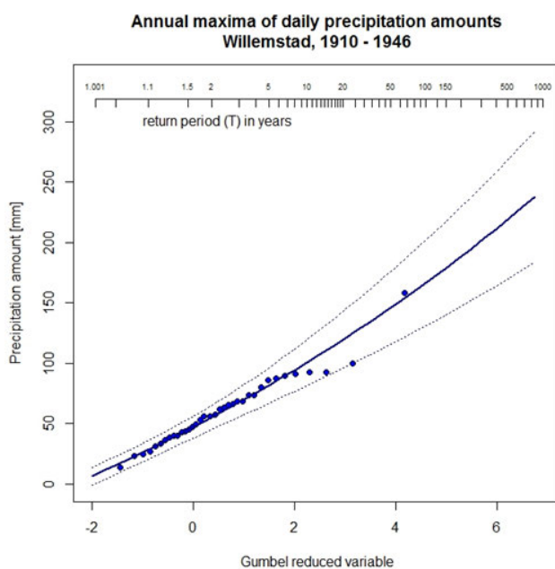
Figuur 33: Neerslagstatistiek opgesteld voor Willemstad Curaçao. Links de extreme waarde verdeling en rechts de neerslaghoeveelheden bij een aantal herhalingstijden. Bron KNMI [17].
