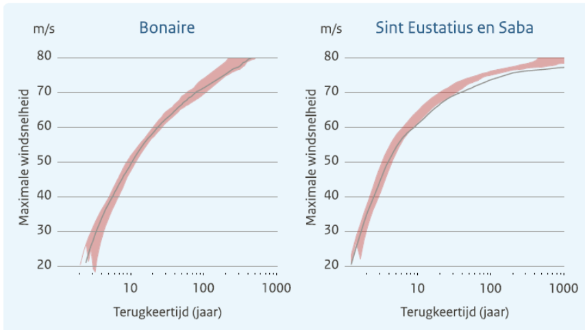
Figuur 28: Herhalingsstijden van een orkaan van de zwaarste categorie binnen 250 km van de BES eilanden. In rood de projectie voor het toekomstige klimaat (2015-2050) bij het hoge uitstootscenario, bron: KNMI'23.
