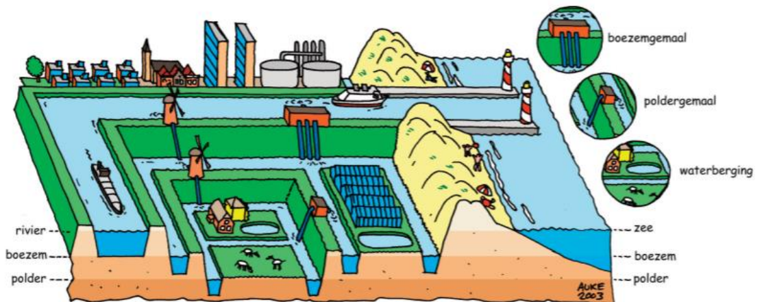
Polder-boezemsysteem
