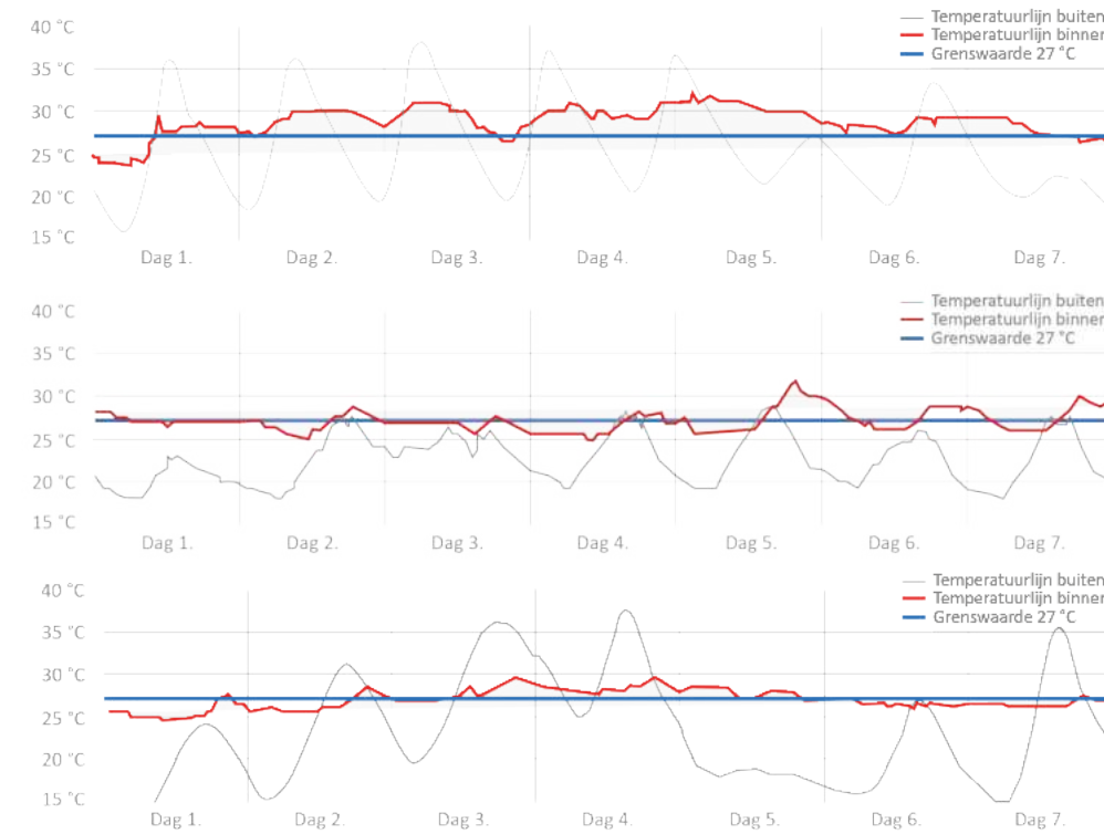
Temperatuurreeks dakverdieping hittegolf. Galerij appartement periode augustus 2022
