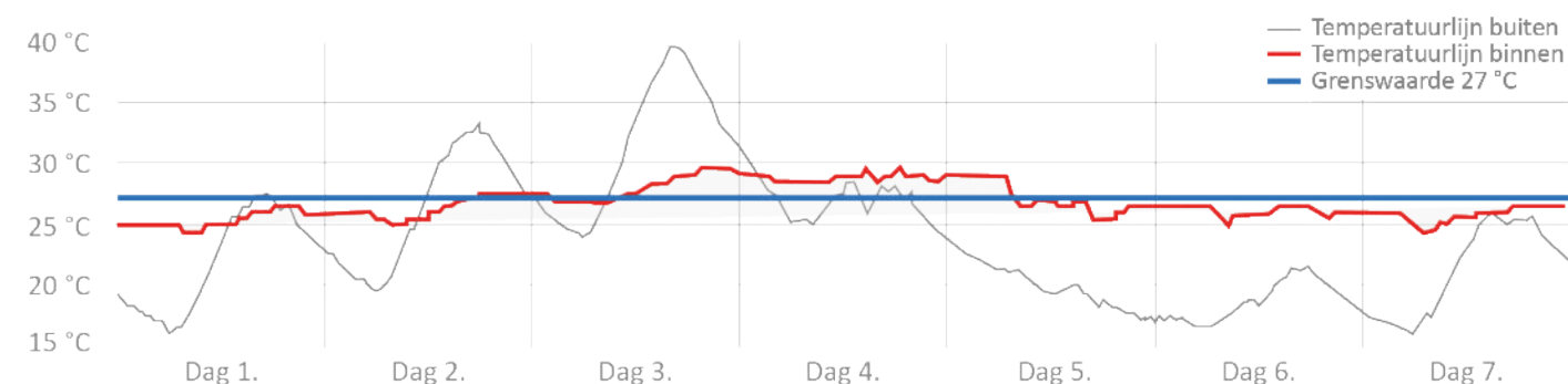
Temperatuurreeks portiekwoning in een hitte-eiland.
