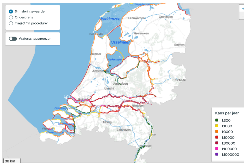
Figuur 6: Ontwerpnormen voor rivierdijken tegen overstromingen (Rijkswaterstaat, n.d.)
